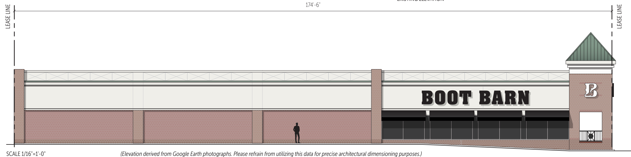
SCALE 1/16"=1'-0"
